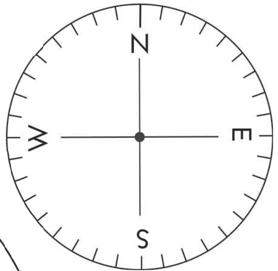
Fig. 13: The horizon disk.
