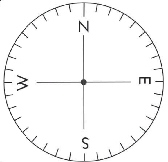
Fig. 5: The horizon disc.
